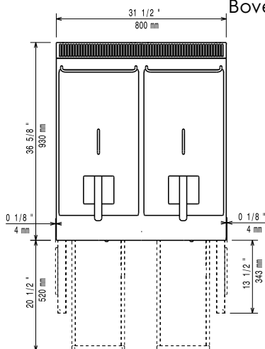
Boven aanzicht
